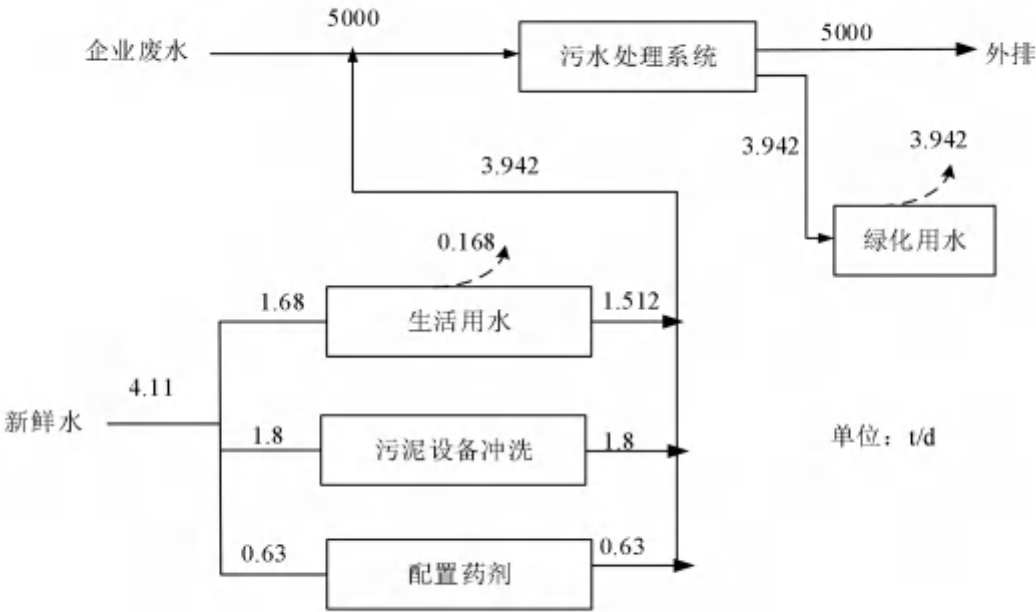
图 2-1 本项目给排水平衡图（单位：m³/d）
